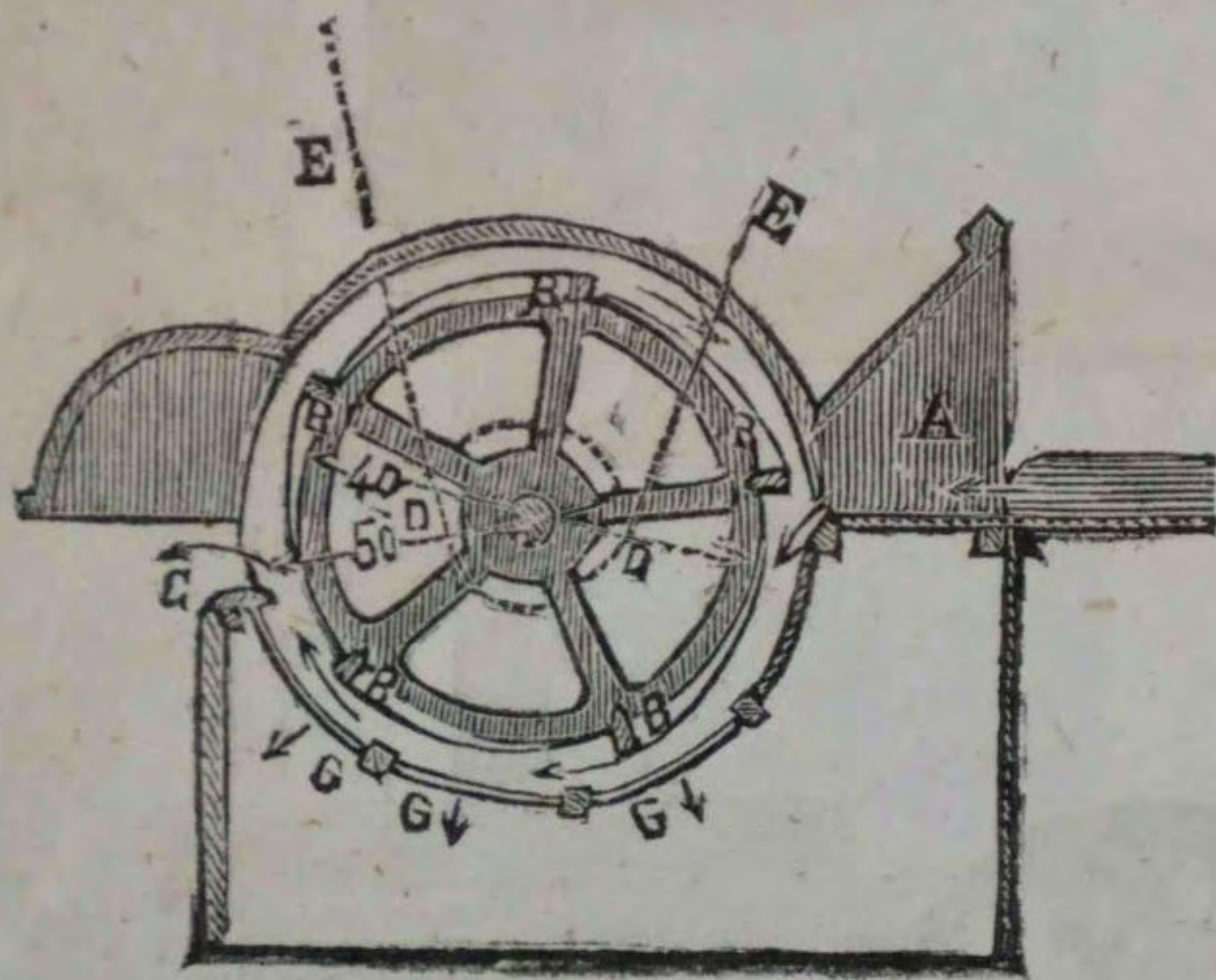
Fig. 113. — Dettaglio di una macchina da battere.
