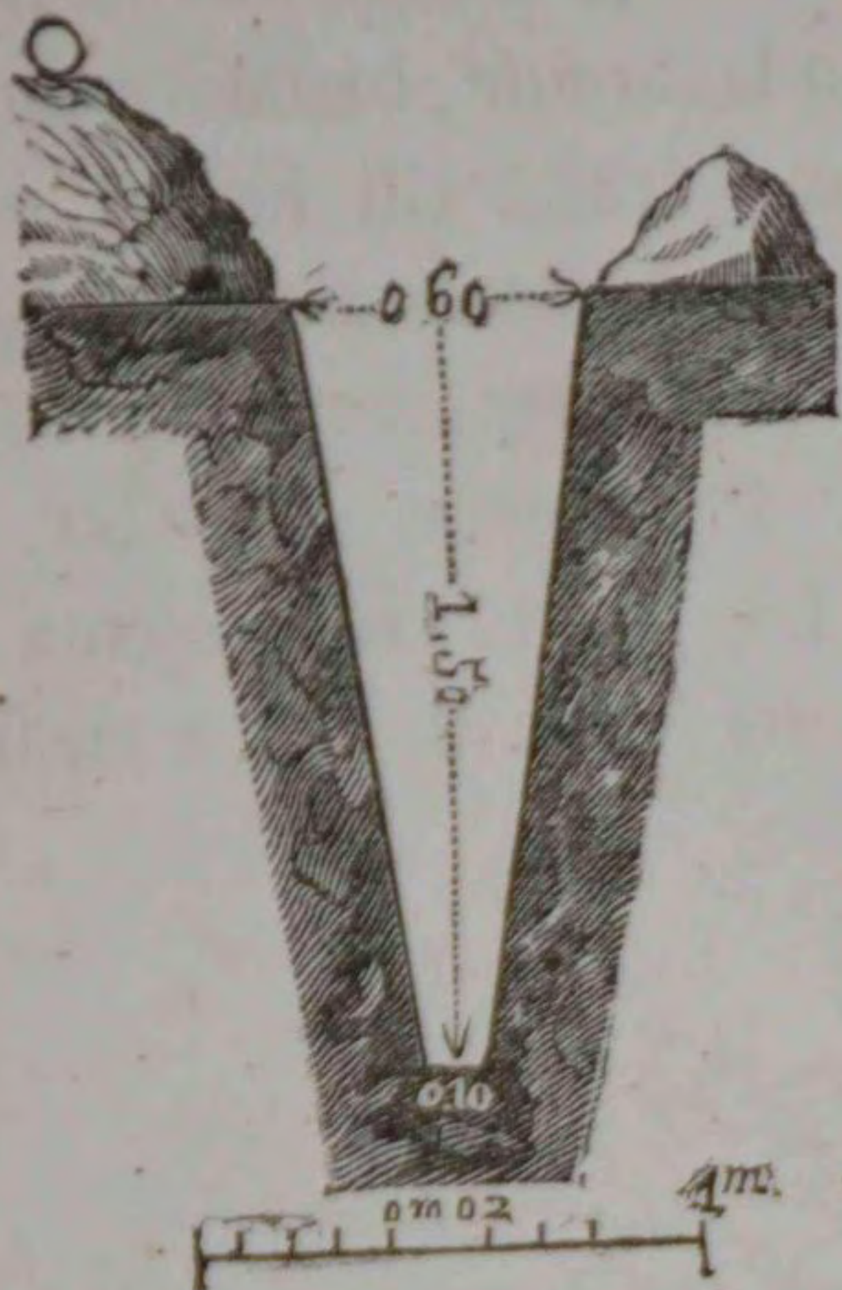
Fig. 14. — Fossa profonda.
