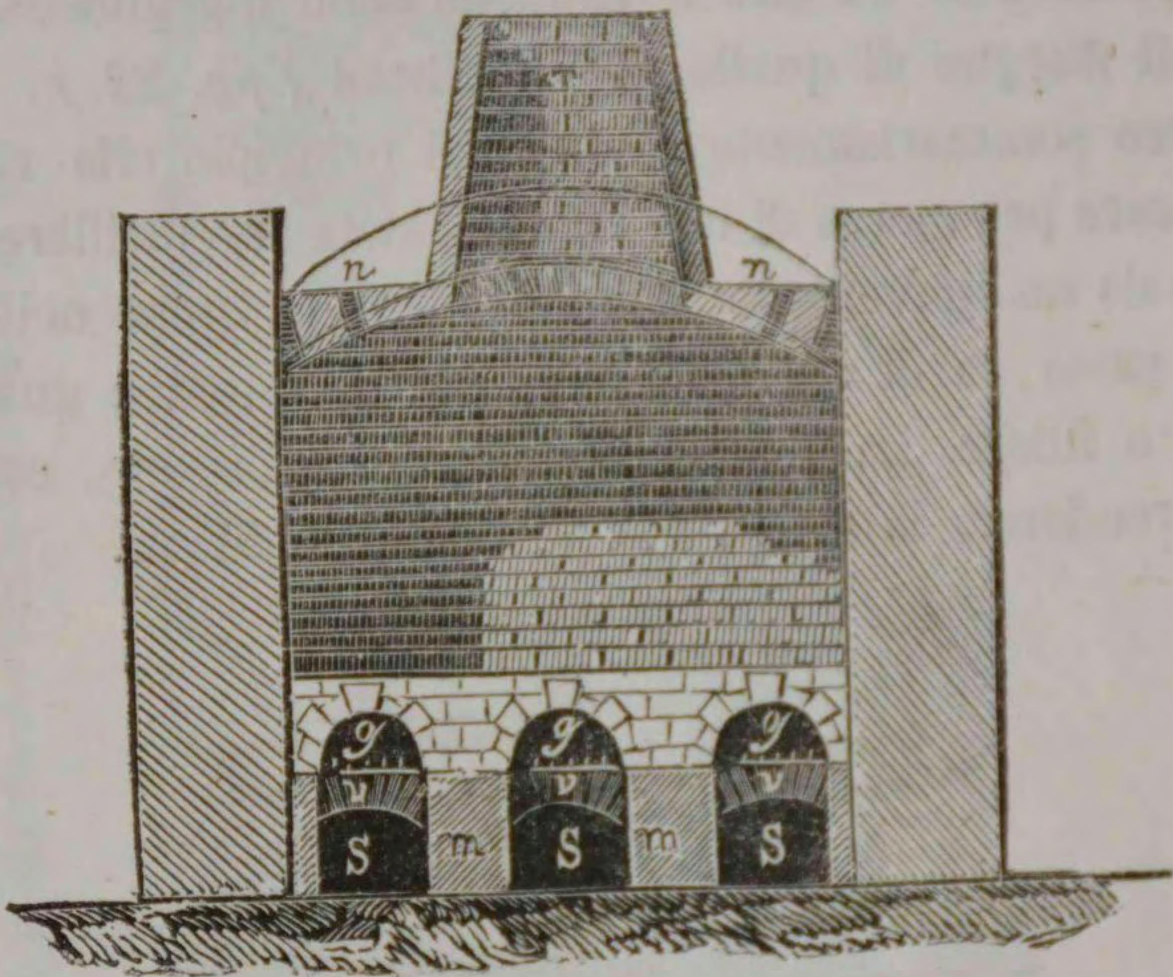
Fig. 24. — Fornace da cannelle.
