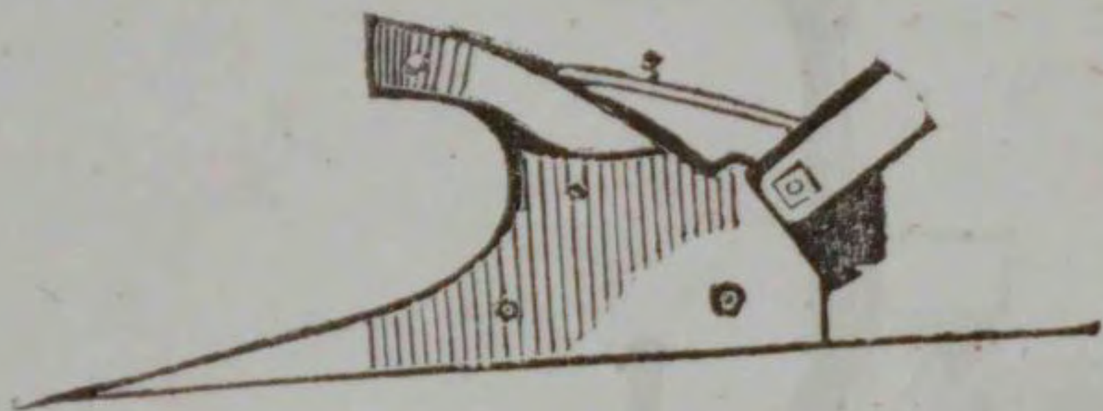
Fig. 29. — Dentale dell'aratro.
