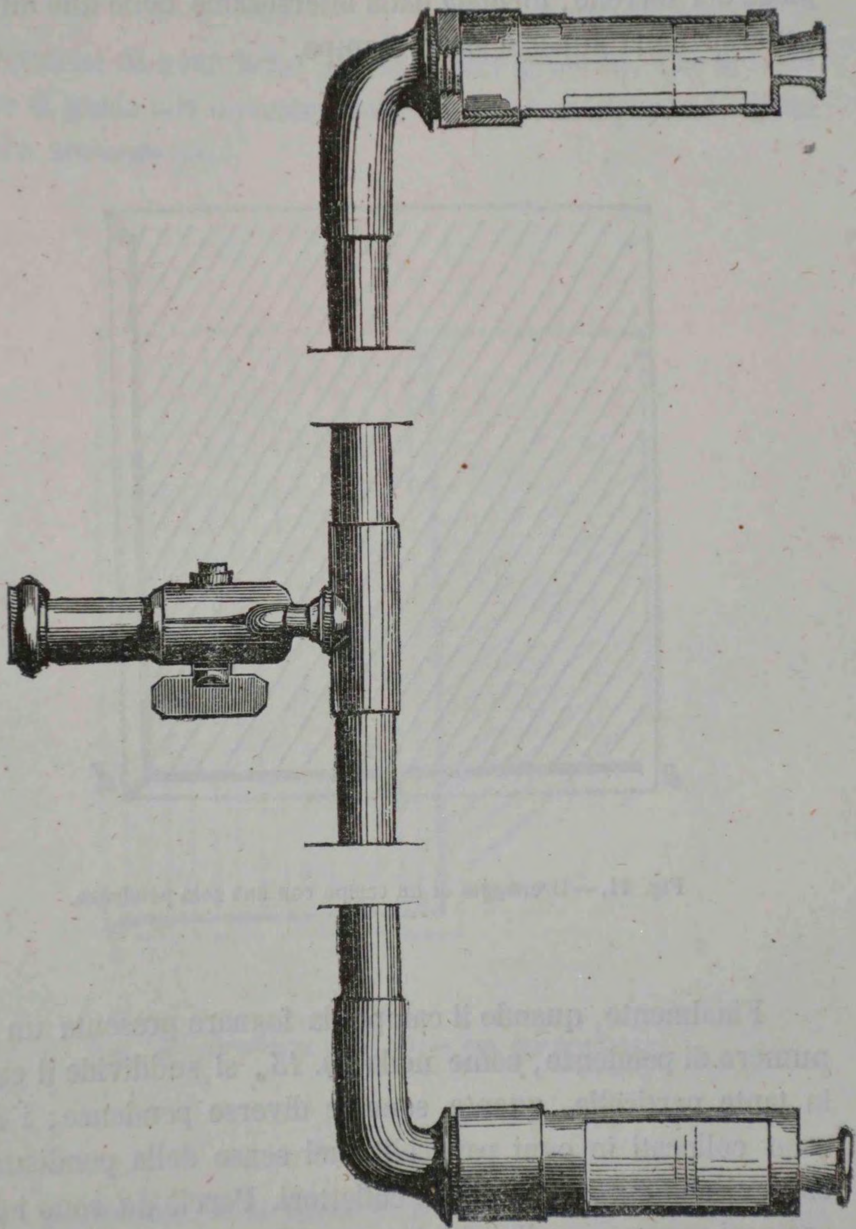
Fig. 10. — Livello a acqua.
