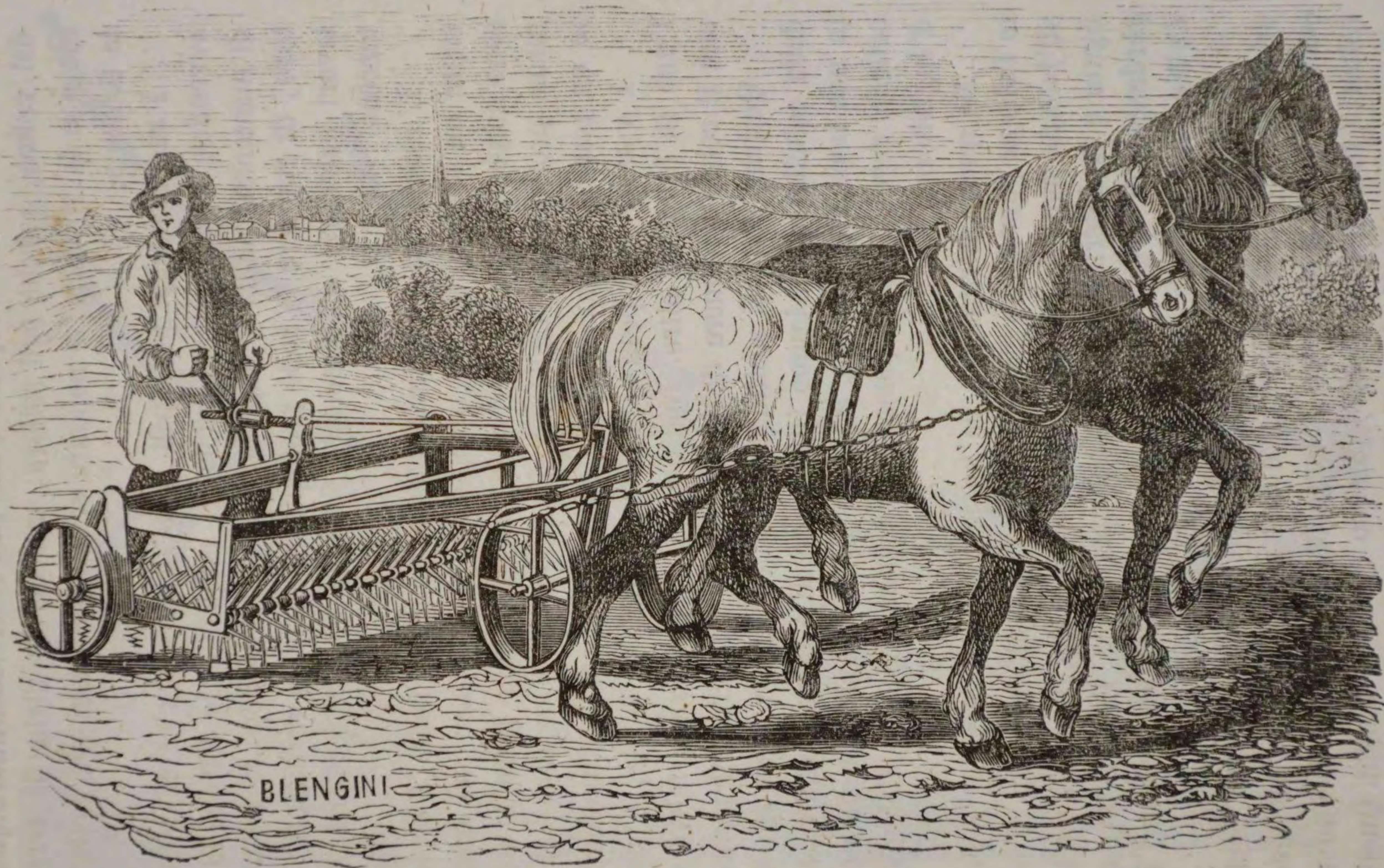
Fig. 44. — Erpice di Norvegia.
