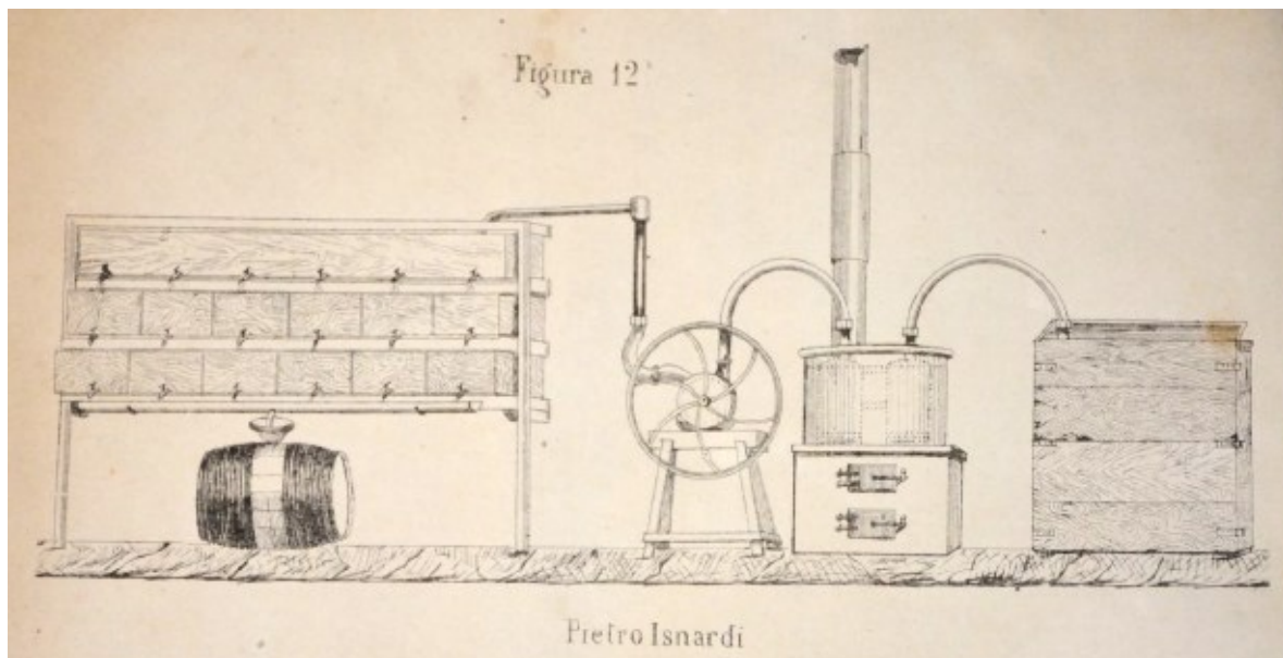
Figura 12: Filtro del Signor Pietro Isnardi di Livorno.
