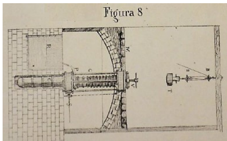
Figura 8: Torchio idrostatico privilegiato.
